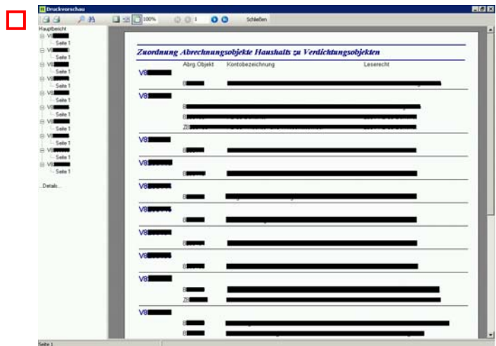
Abb. 4-1: Druckvorschau Report
